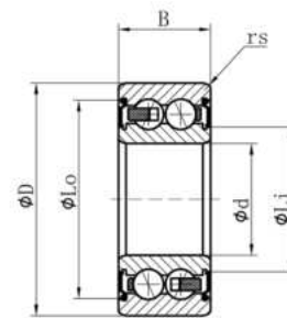
Shielded (ZZ)
